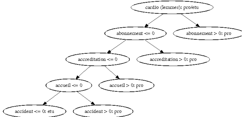
Figure 2 : Arbre de décision pour la distinction entre les documents professionnels et étudiants. La distinction automatique exploite les informations lexicales : occurrences des lemmes.
