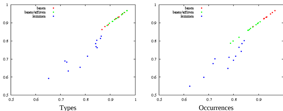
Figure 1 : Performance des méthodes automatiques par apprentissage supervisé dans la distinction des types de documents selon leur technicité.
